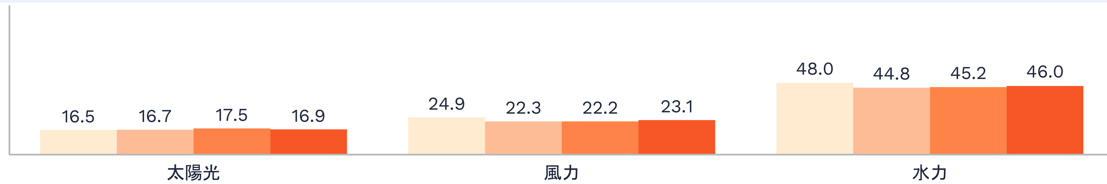
年別・断続的な再生可能エネルギー別の年間設備利用率 (%)
