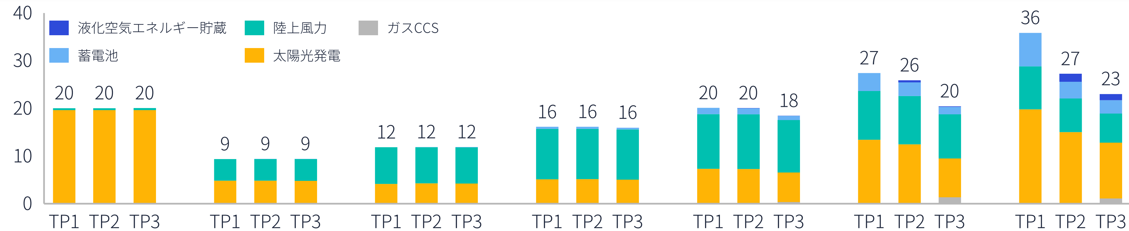
グリーンフィールド発電 - 全国合計 (TWh) 1
