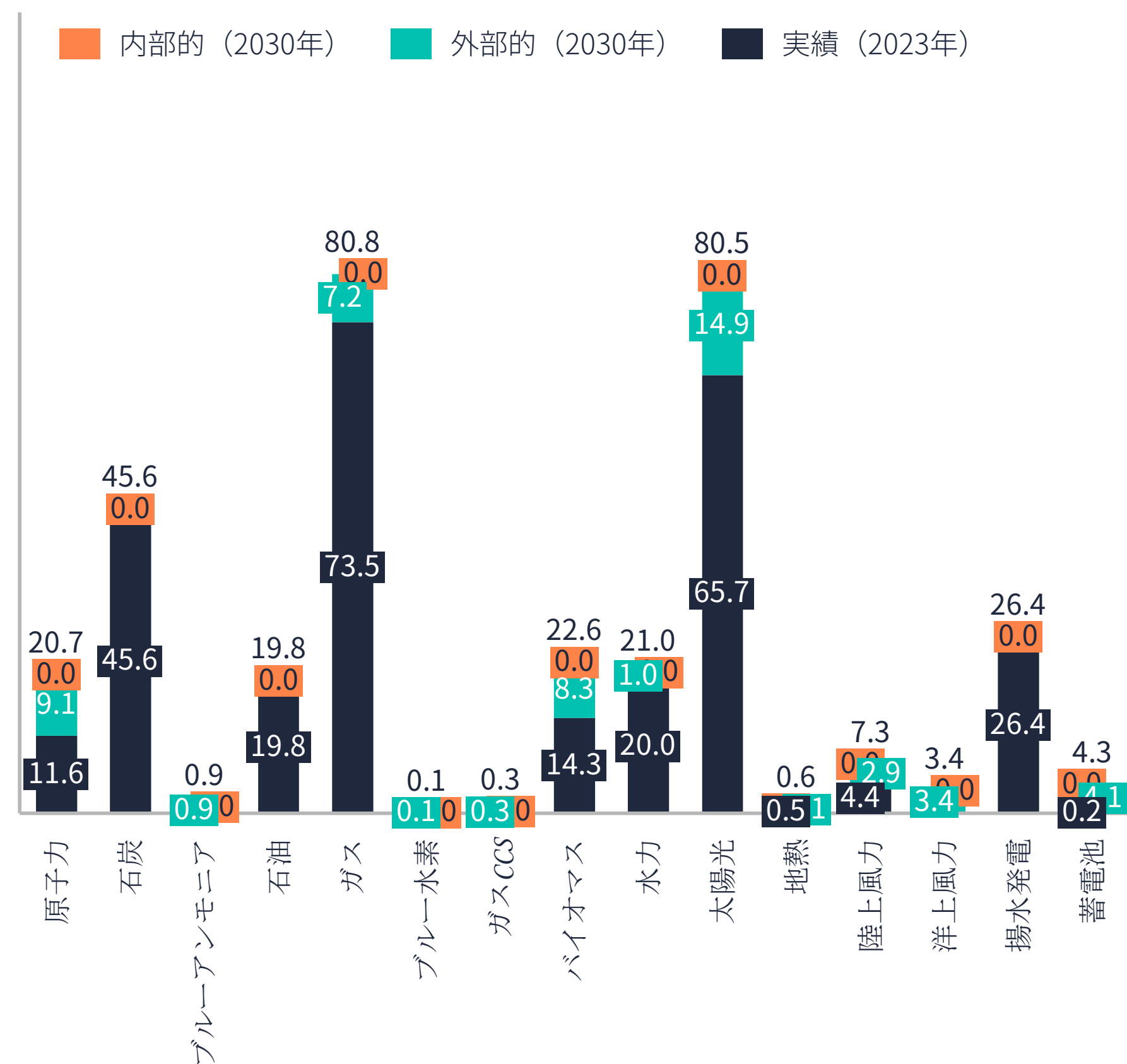
施設容量 2 (GW)
