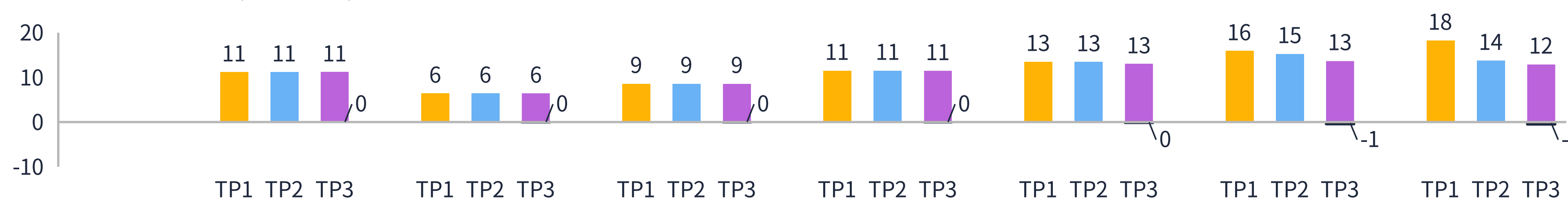
全国的な排出削減(MtCO 2 e)
