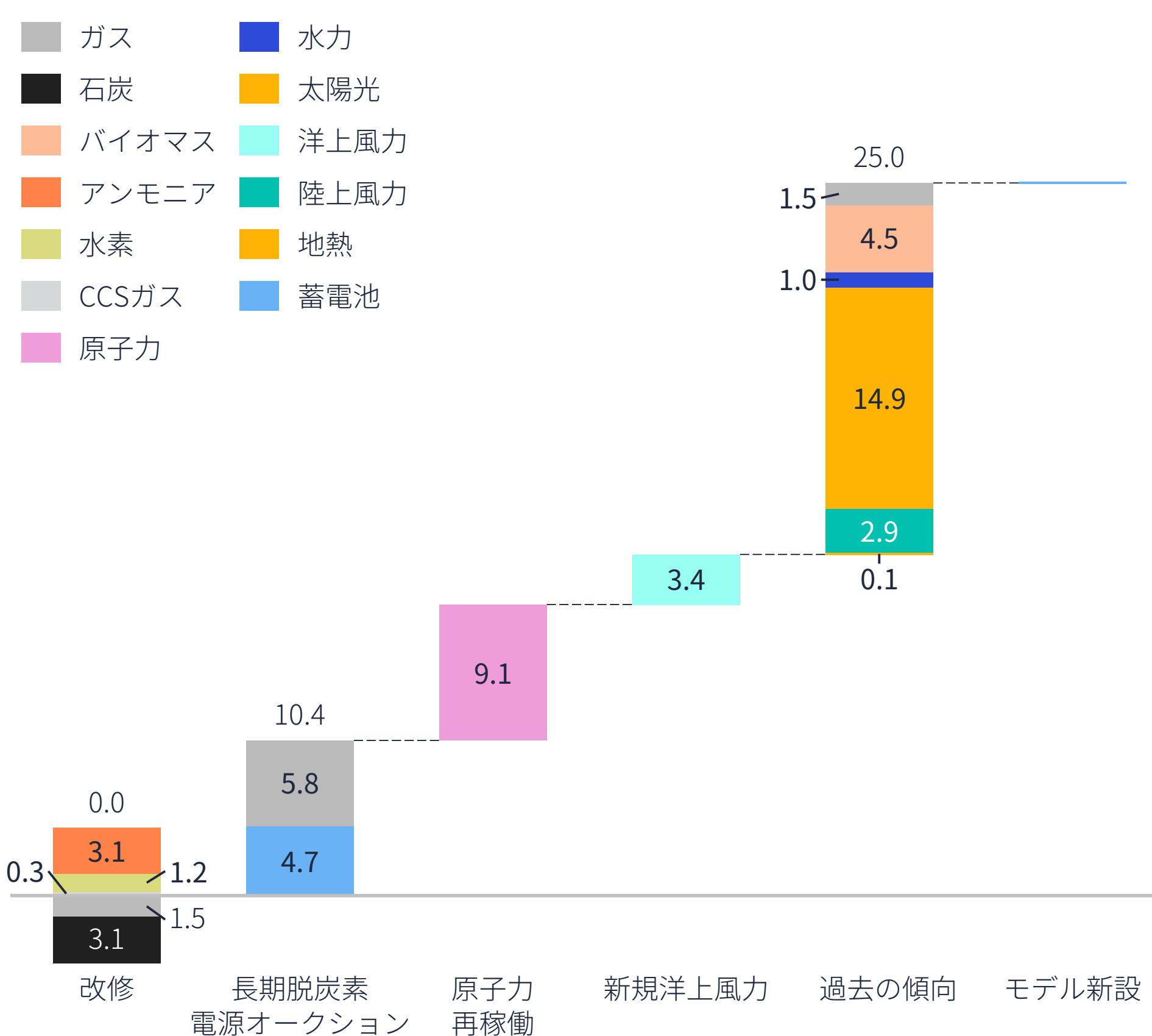
2030年の外部的容量の内訳 (GW)
