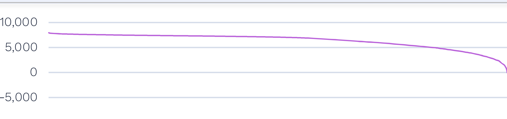
中部向け連系線の降順空き容量 4 (MW)
