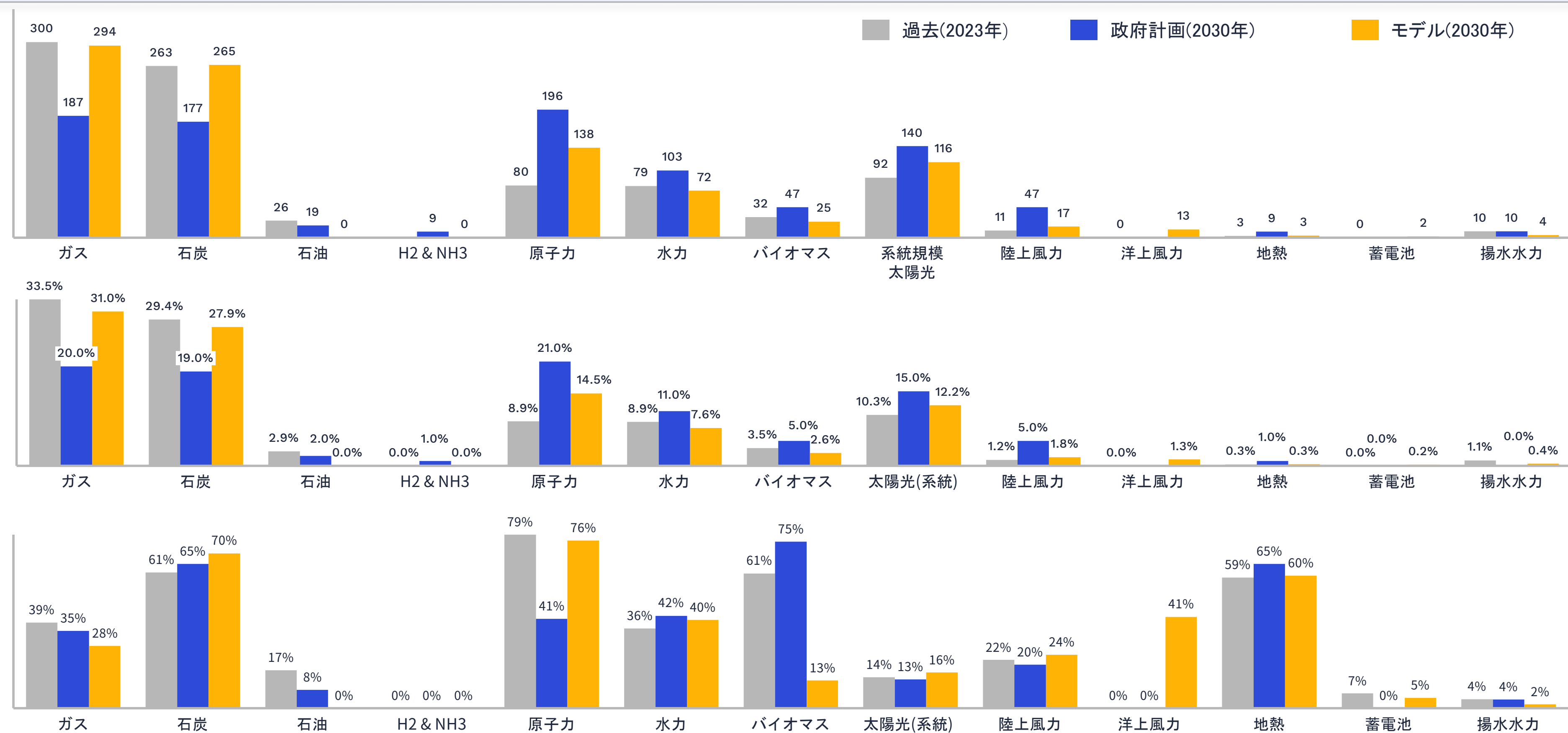
発電方式およびシナリオ別の発電（TWh、総発電量に占める割合(%)、% of year 1 ）
