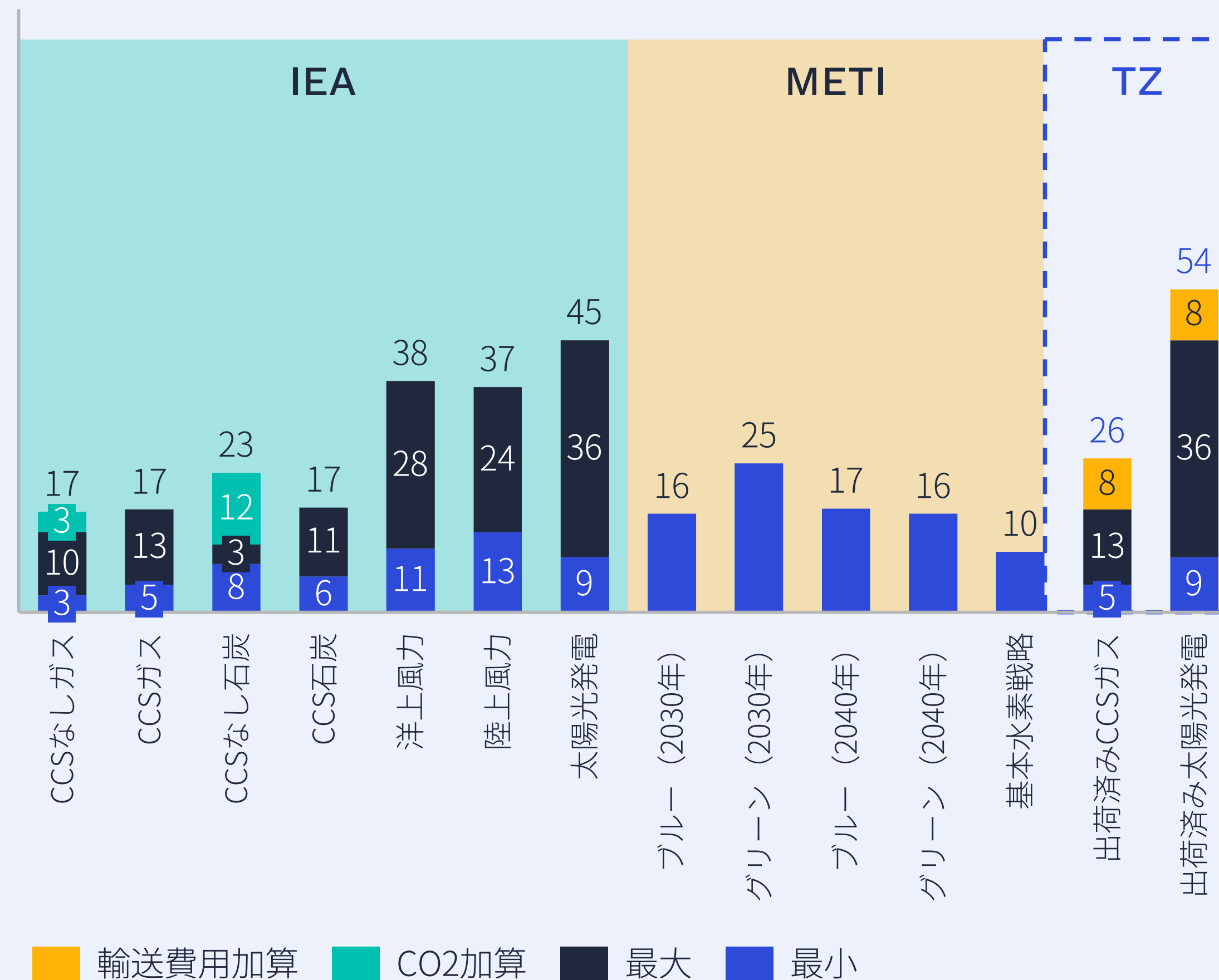
発生源別水素価格 (千円/MWh)
