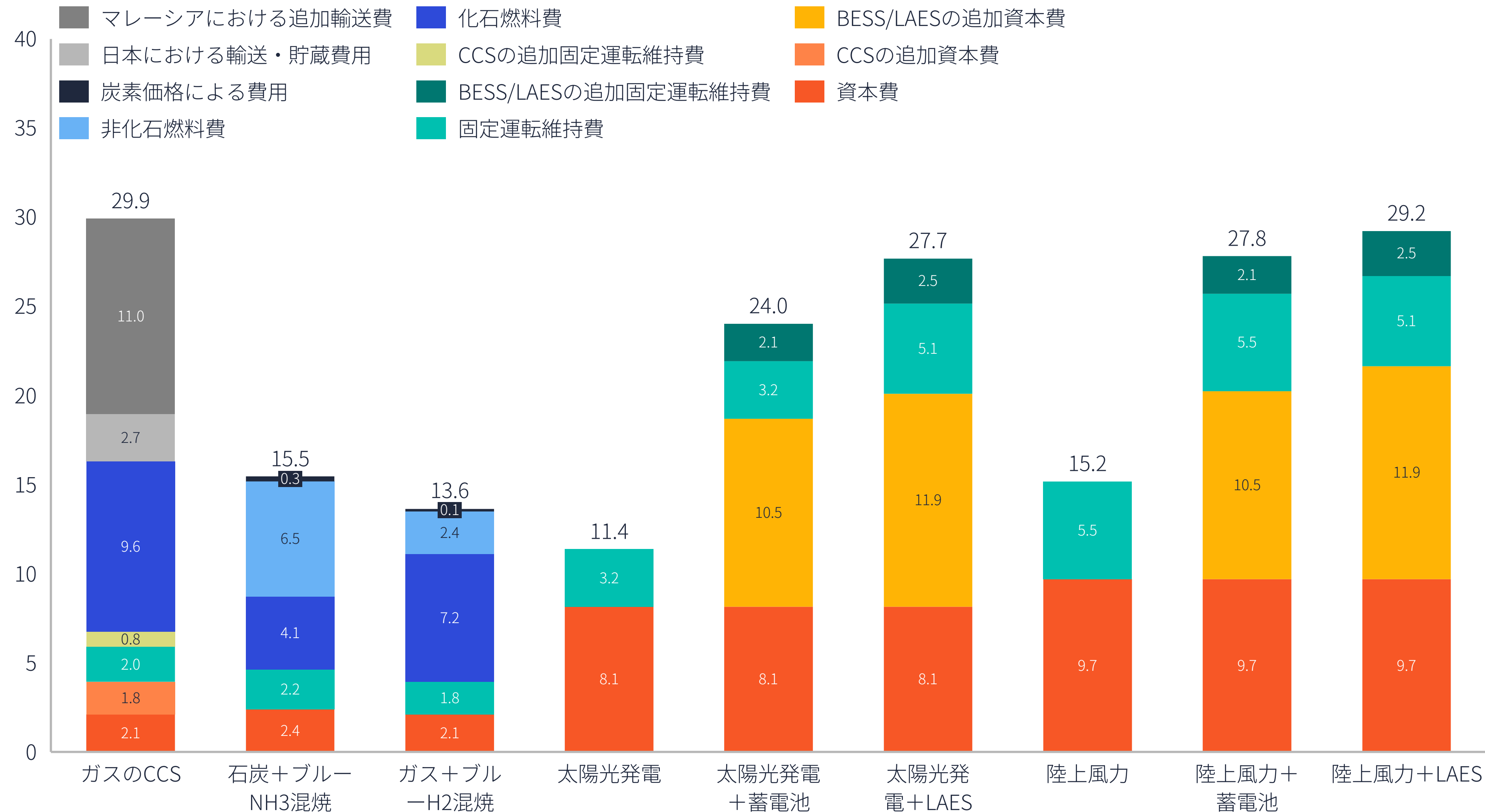
発電方式別LCOE 1 (千円/MWh)
