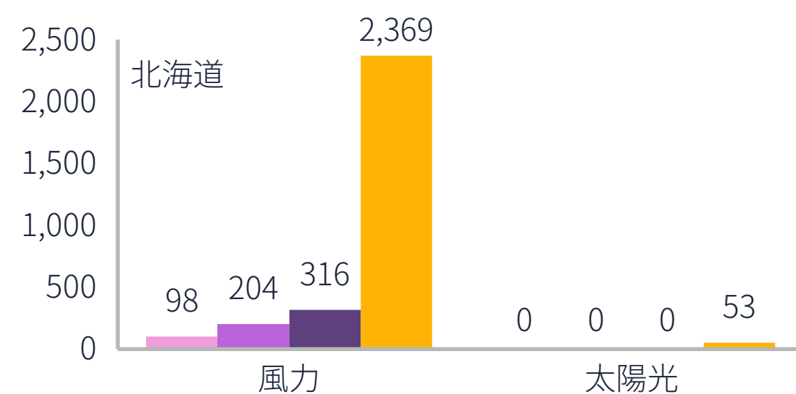
現在の参照値に対して必要な新增設(MW) 2
