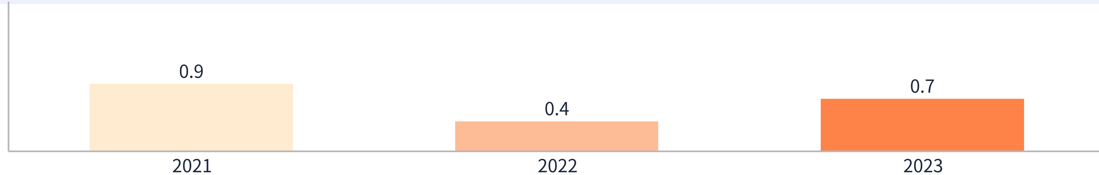
年別・断続的な再生可能エネルギー別の発電量 (TWh)
