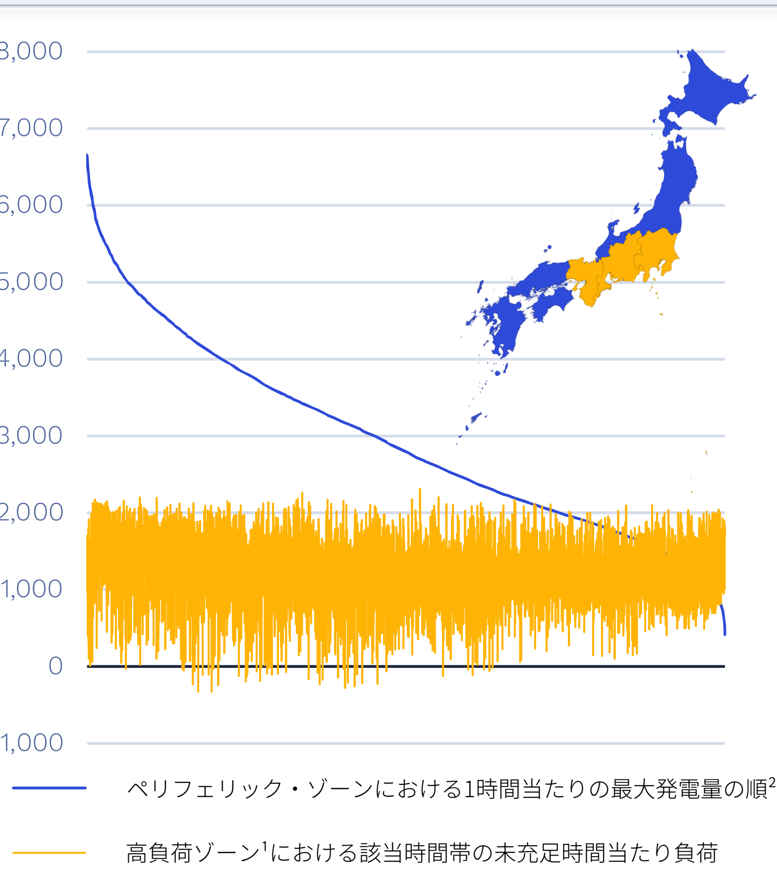
高負荷エリアへの供給ポテンシャル（MW）
