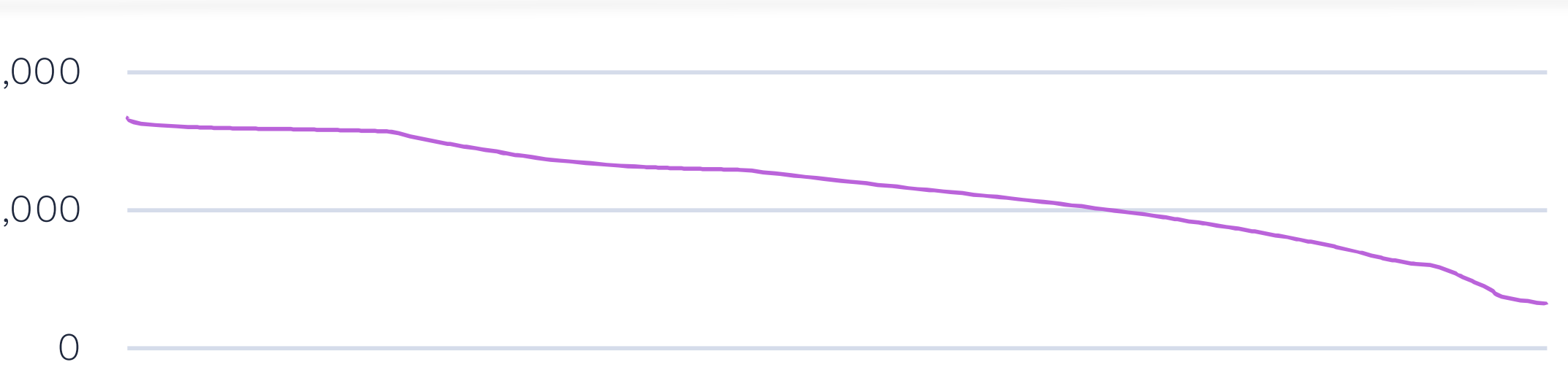
関西向け連系線の降順空き容量 5 (MW)
